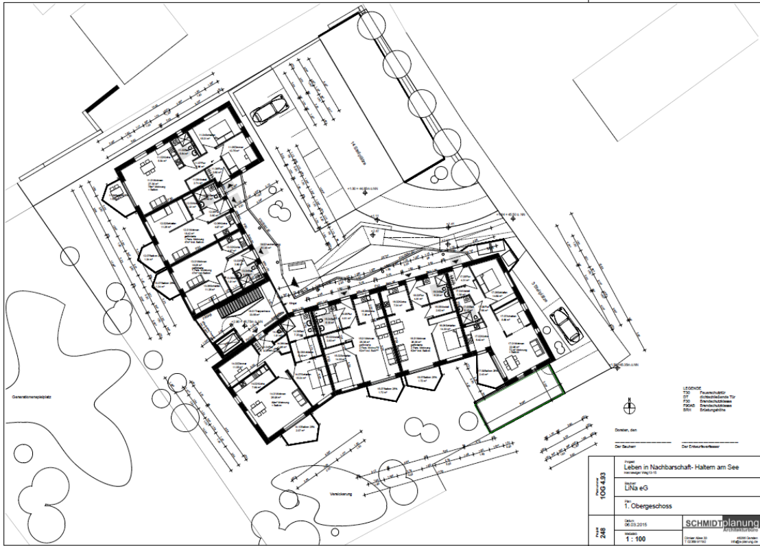
Grundriss des ersten und zweiten Obergeschosses
